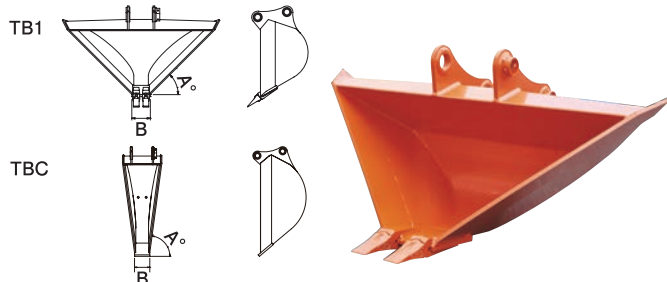
■梯形(三角)バケット TB5 仕様表
