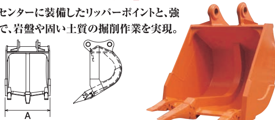
■リッパースタンプバケット 仕様表
